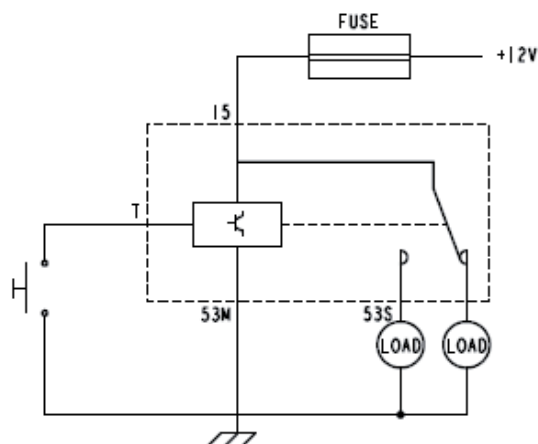
SCHEMA DI COLLEGAMENTO CIRCUIT DIAGRAM
