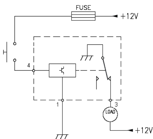
SCHEMA DI COLLEGAMENTO CIRCUIT DIAGRAM
