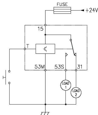
SCHEMA DI COLLEGAMENTO CIRCUIT DIAGRAM
