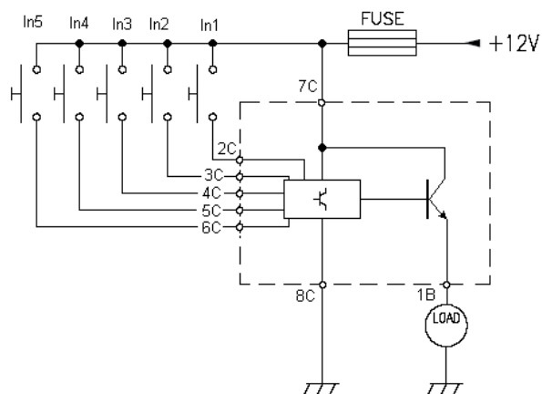
SCHEMA DI COLLEGAMENTO CIRCUIT DIAGRAM
