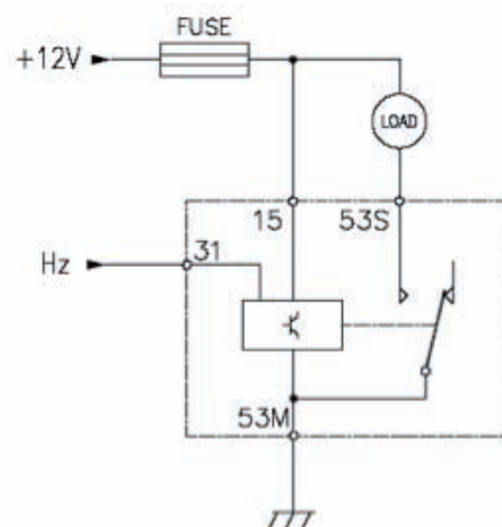
SCHEMA DI COLLEGAMENTO CIRCUIT DIAGRAM
