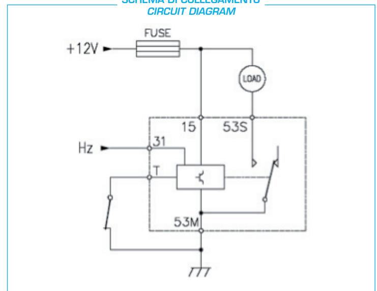
SCHEMA DI COLLEGAMENTO CIRCUIT DIAGRAM
