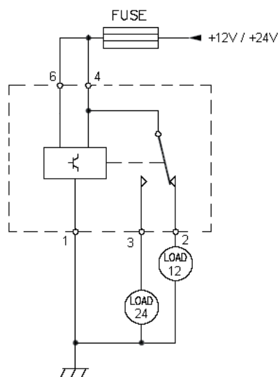
SCHEMA DI COLLEGAMENTO CIRCUIT DIAGRAM
