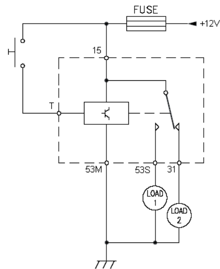
SCHEMA DI COLLEGAMENTO CIRCUIT DIAGRAM
