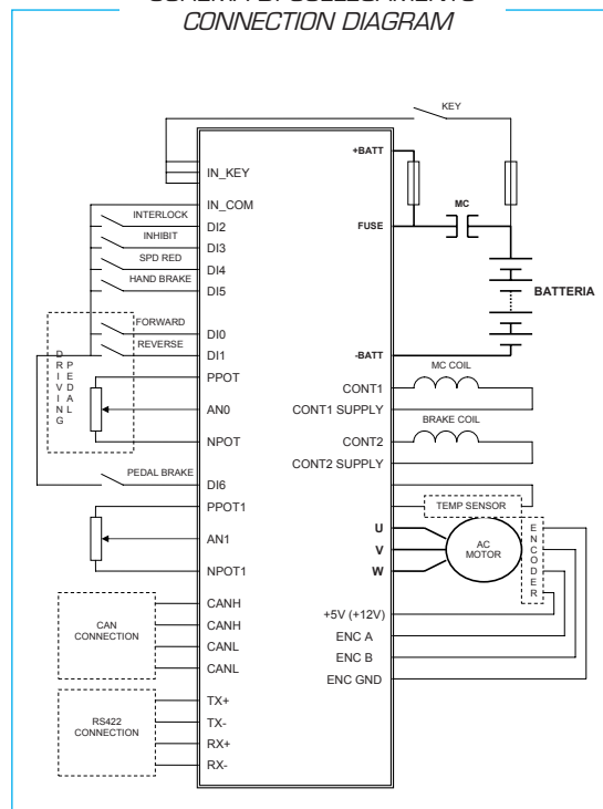
SCHEMA DI COLLEGAMENTO CONNECTION DIAGRAM
