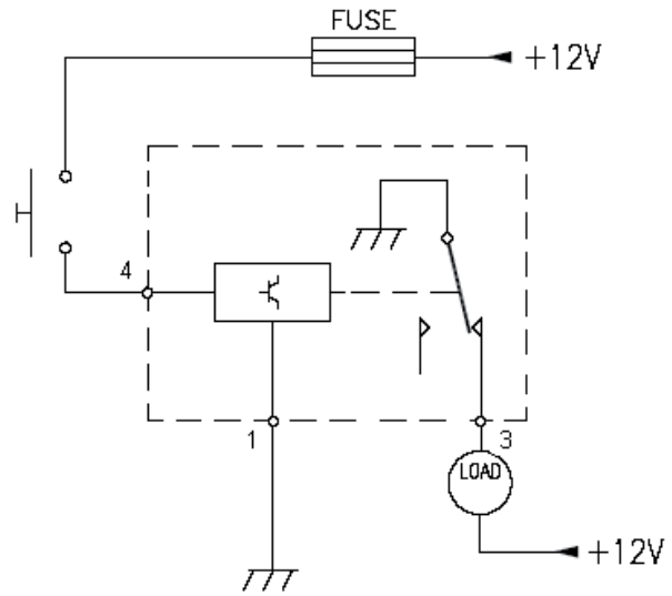
SCHEMA DI COLLEGAMENTO CIRCUIT DIAGRAM
