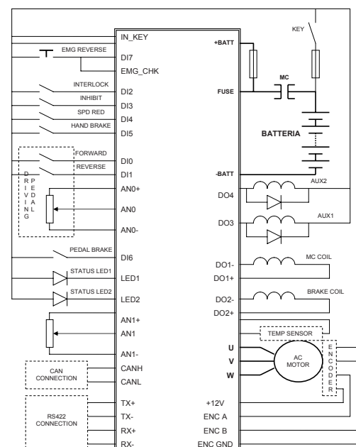
SCHEMA DI COLLEGAMENTO CONNECTION DIAGRAM
