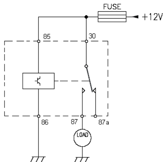
SCHEMA DI COLLEGAMENTO CIRCUIT DIAGRAM
