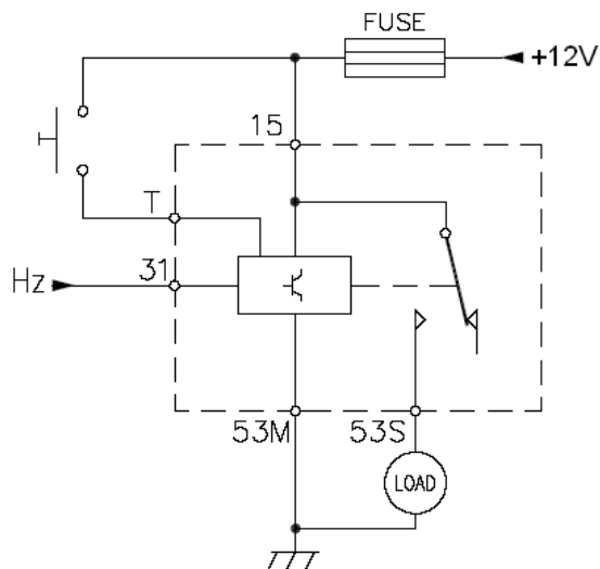
SCHEMA DI COLLEGAMENTO CIRCUIT DIAGRAM
