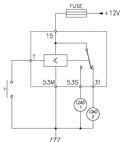
SCHEMA DI COLLEGAMENTO CIRCUIT DIAGRAM
