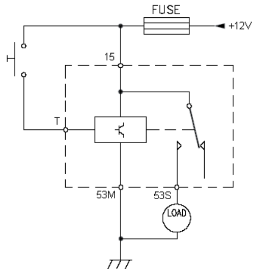
SCHEMA DI COLLEGAMENTO CIRCUIT DIAGRAM
