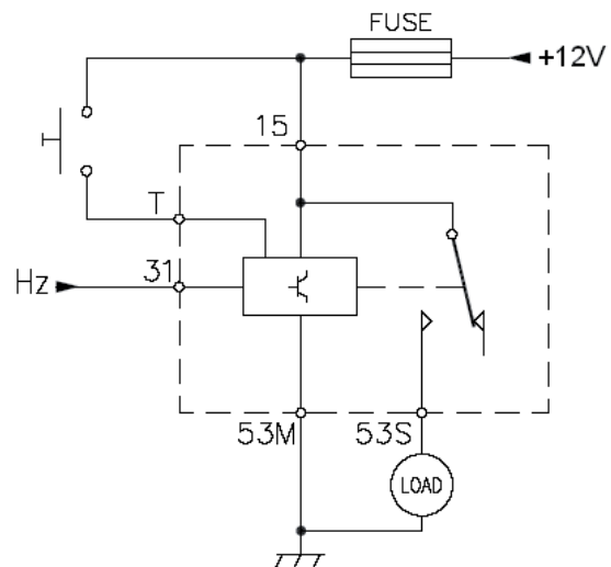
SCHEMA DI COLLEGAMENTO CIRCUIT DIAGRAM
