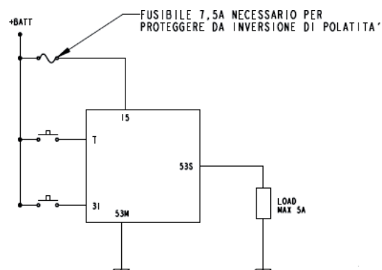
SCHEMA DI COLLEGAMENTO CIRCUIT DIAGRAM
