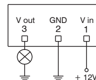
SCHEMA DI COLLEGAMENTO CIRCUIT DIAGRAM
