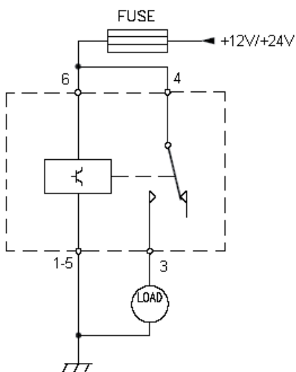
SCHEMA DI COLLEGAMENTO CIRCUIT DIAGRAM
