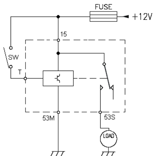
SCHEMA DI COLLEGAMENTO CIRCUIT DIAGRAM
