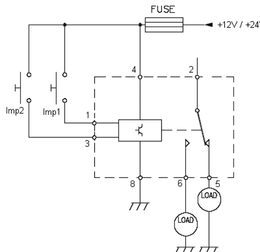
SCHEMA DI COLLEGAMENTO CIRCUIT DIAGRAM
