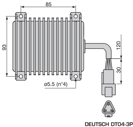
DEUTSCH DT04-3P
