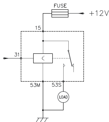
SCHEMA DI COLLEGAMENTO CIRCUIT DIAGRAM
